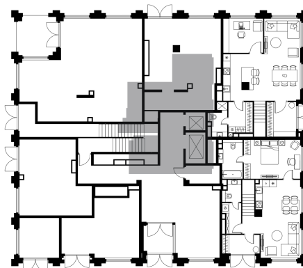
План этажа (2 этаж)
