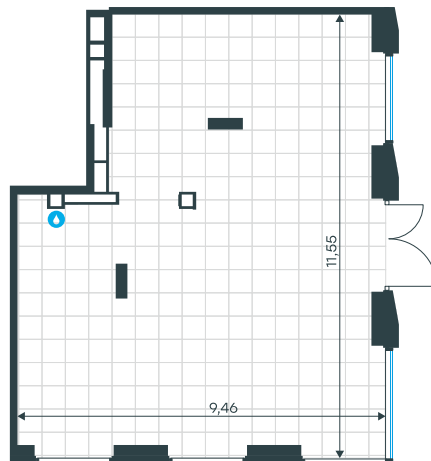
План этажа
