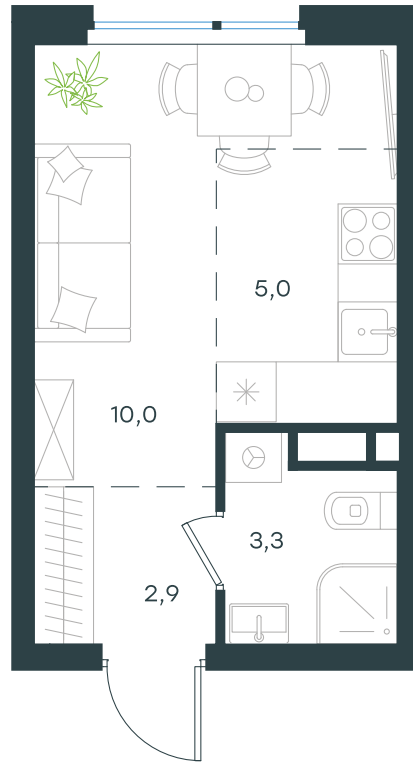
План этажа
