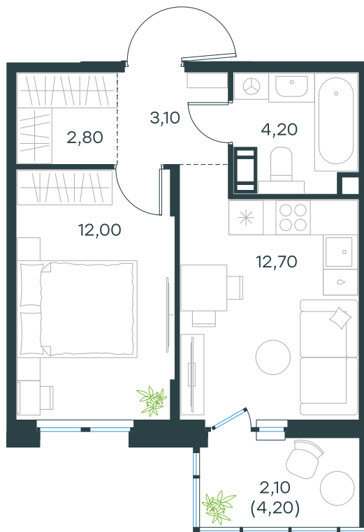
План этажа
