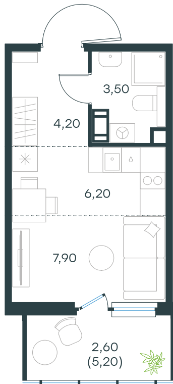
План этажа
