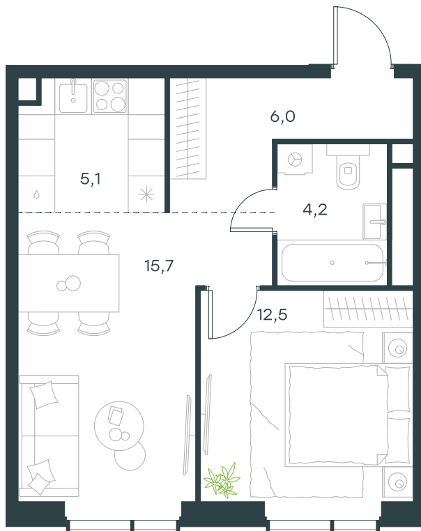
План этажа
