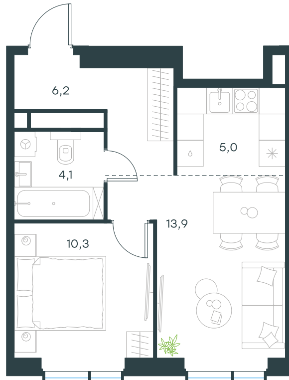
План этажа
