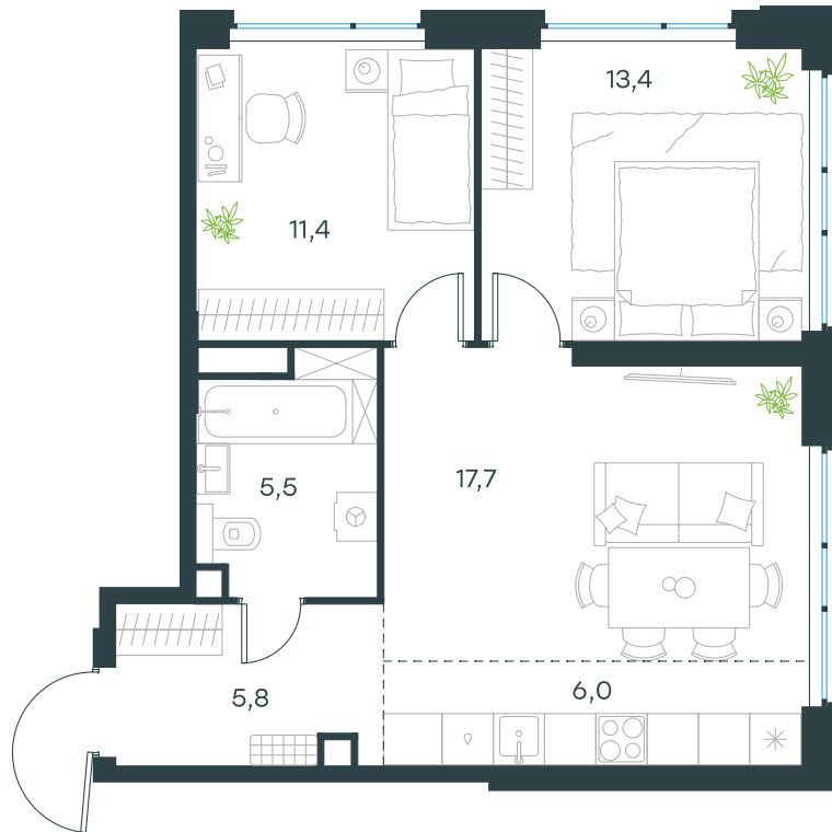
План этажа
