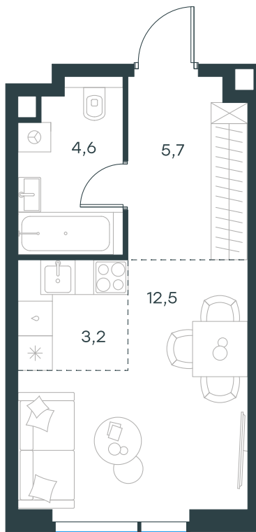
План этажа
