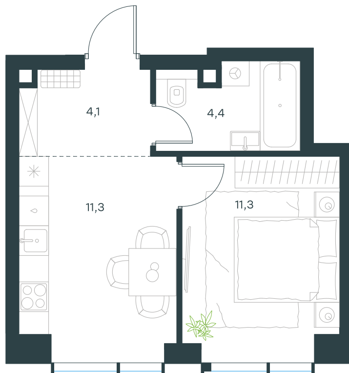
План этажа
