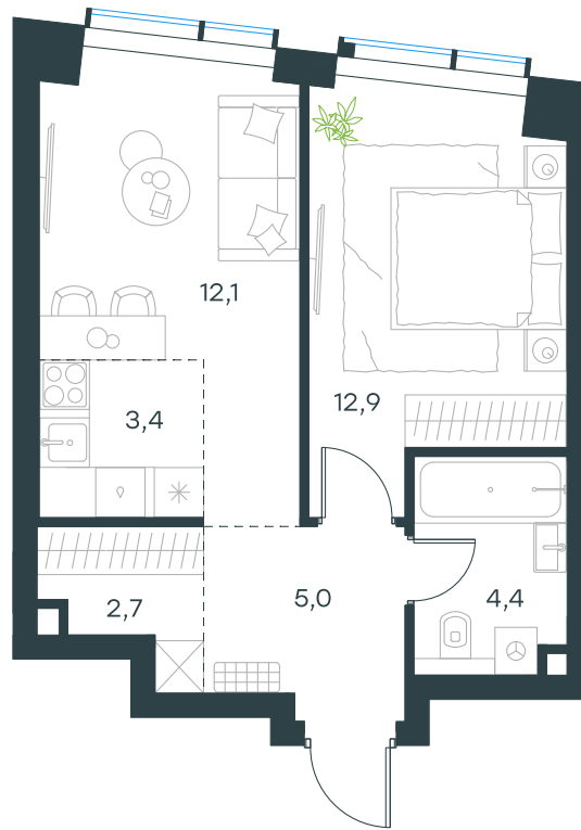
План этажа
