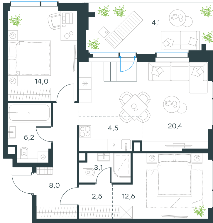
План этажа
