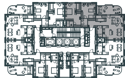
План этажа (1 этаж)
