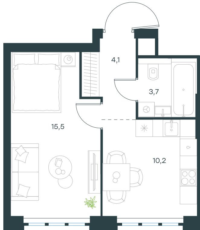
План этажа
