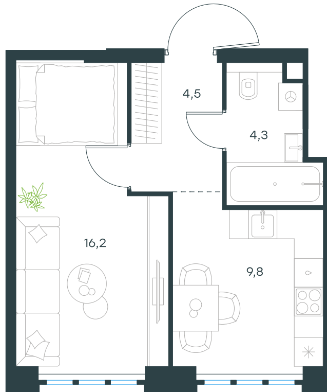
План этажа
