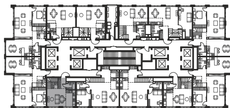
План этажа (1 этаж)
