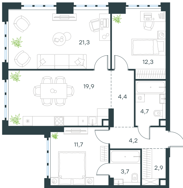
План этажа
