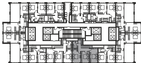
План этажа (2 этаж)
