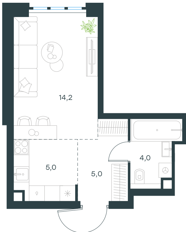
План этажа
