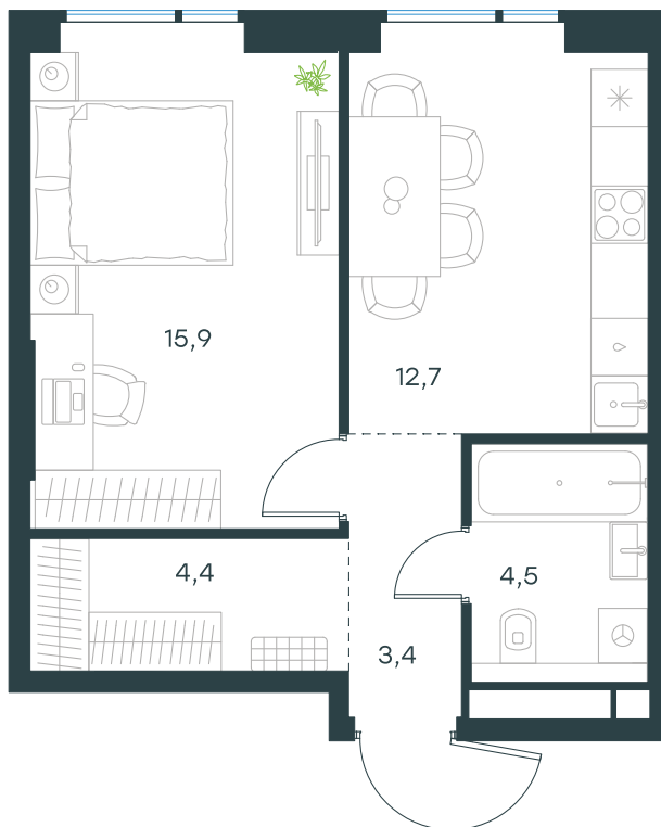
План этажа
