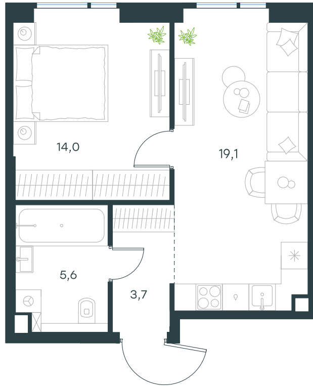
План этажа
