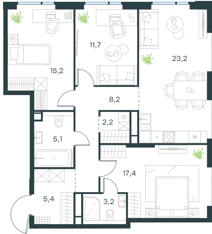
План этажа
