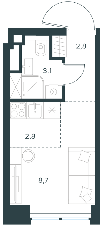
План этажа
