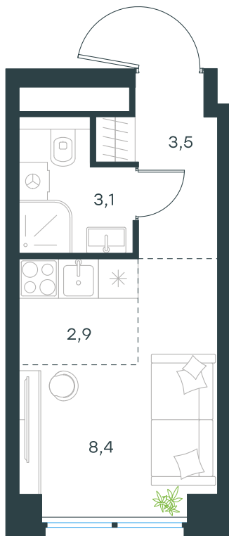
План этажа
