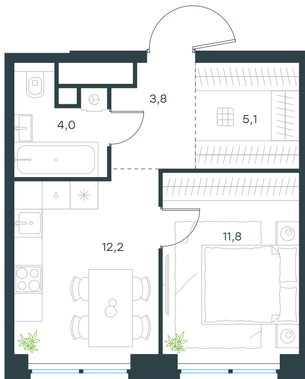
План этажа
