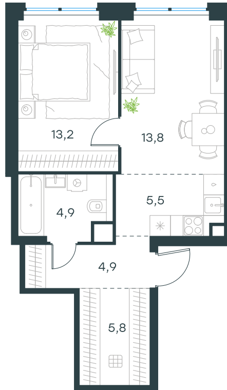
План этажа
